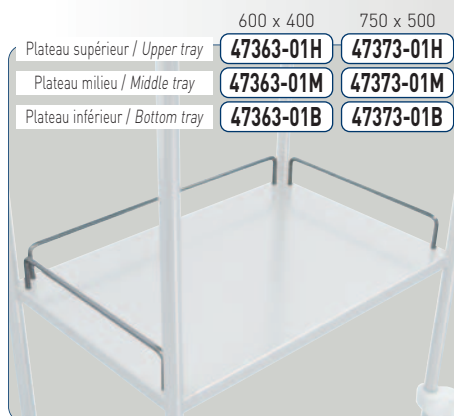
Galerie 3 côtés 3 guard rails
